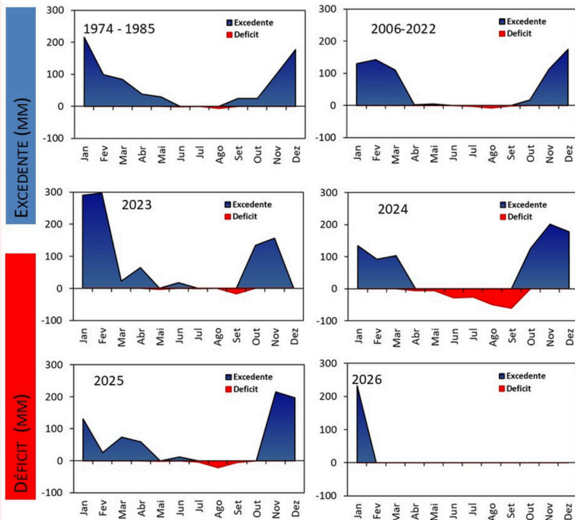
Figura 8: Balanço hídrico mensal (THORNTHWAIT E MATHER, 1955) no período de 1974-1985, 2006-2022, para os anos de 2023, 2024, 2025 e 2026 para a região do Sul de Minas, Muzambinho.
