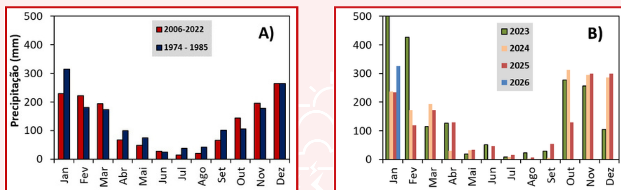
Figura 3: Precipitação pluviométrica média mensal (mm) das médias históricas de 1974-1985, 2006-2022 (A) e dos anos 2023, 2024, 2025 e 2026 (B) para a região do Sul de Minas, Muzambinho.
