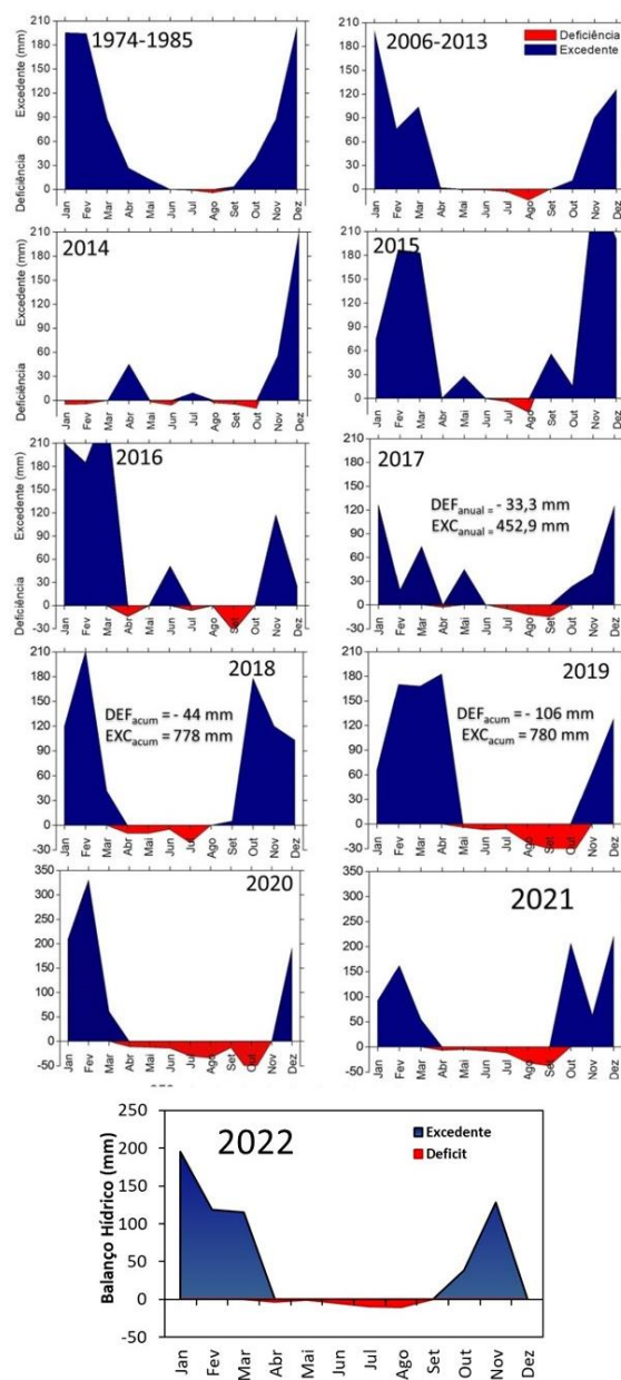
Figura 8: Balanço hídrico mensal sequencial (THORNTHWAITTE E MATHER, 1955) no período de 1974-1985, 2006-2013, para os anos de 2014, 2015, 2016, 2017, 2018, 2019, 2020, 2021 e 2022 para a região do Sul de Minas, Muzambinho.
